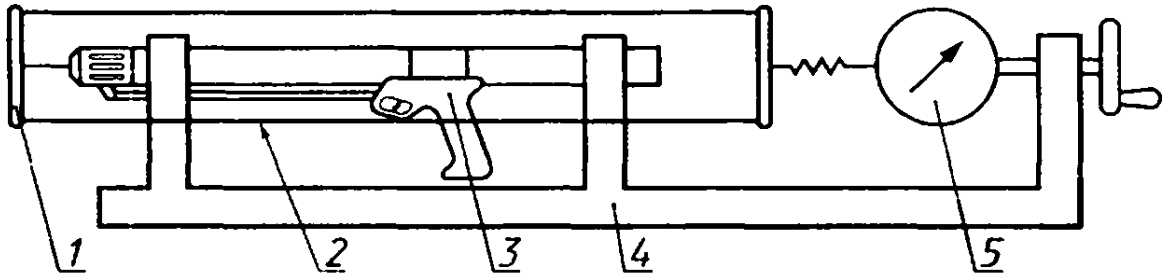
1 - ручка для зарядания, 2 - трос, 3 - оружие, 4 - приспособление, 5 - динамометр
