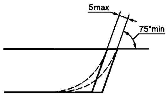
Рисунок 2 — Угол схождения обуха и лезвия клинка
